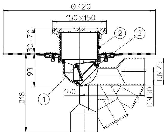
Рис. 1. Трап для балконов и террас HL81GH.
