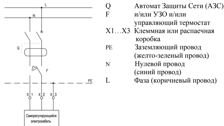
Рис. 5. Схема подключения электрообогрева кровельной воронки HL64.1BH к электрической сети.
