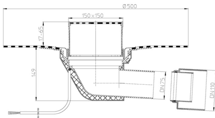
Рис. 1. Кровельная воронка HL64.1ВН.
