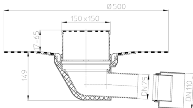
Рис. 1. Кровельная воронка HL64BH.
