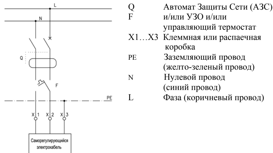
Рис. 5. Схема подключения электрообогрева кровельной воронки HL64.1B к электрической сети.
