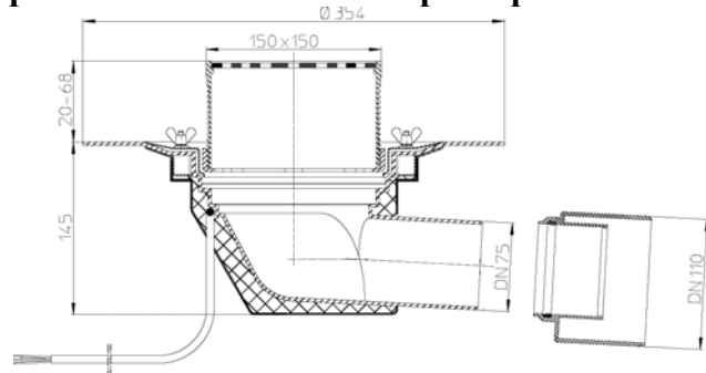
Рис. 1. Кровельная воронка HL64.1В.
