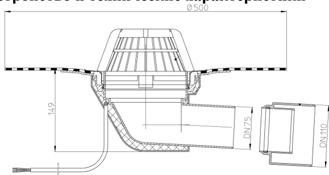
Рис. 1. Кровельная воронка HL64.1H.
