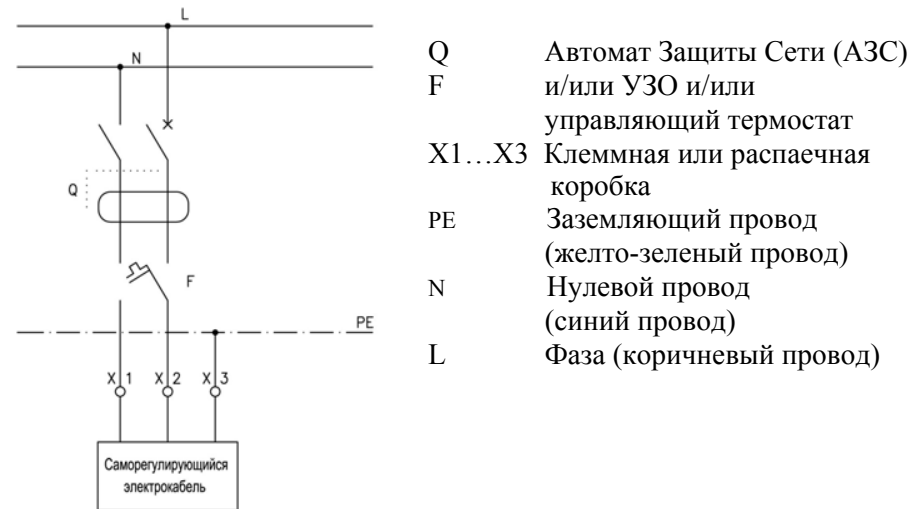
Рис. 5. Схема подключения электрообогрева кровельной воронки HL64.1H к электрической сети.
