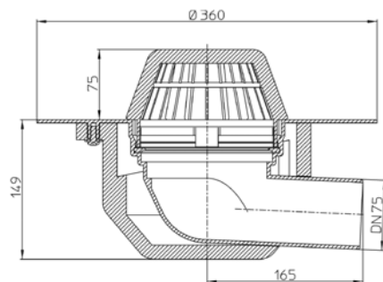
Рис. 1. Кровельная воронка HL64F/7.
