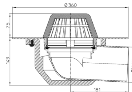
Рис. 2. Кровельная воронка HL64F/1.
