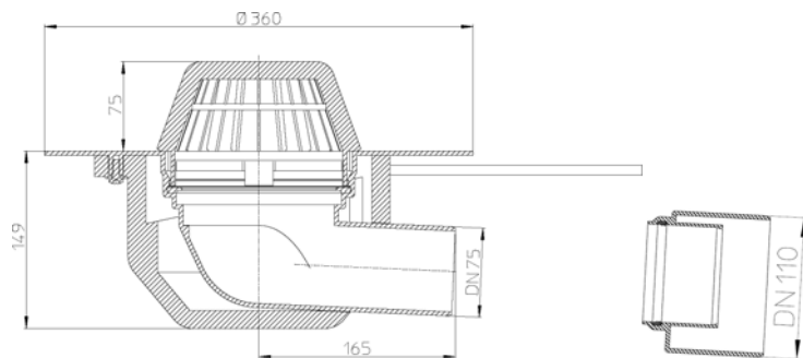
Рис. 1. Кровельная воронка HL64.1P.
