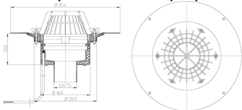
Рис. 1. Кровельная воронка HL62.1/7.
