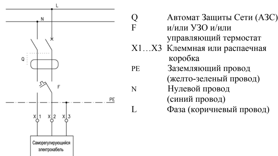
Рис. 5. Схема подключения электрообогрева кровельной воронки HL62.1 к электрической сети.
