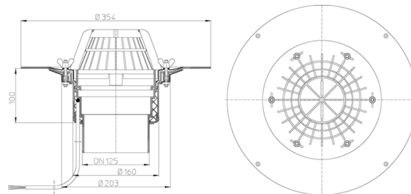
Рис. 3. Кровельная воронка HL62.1/2.
