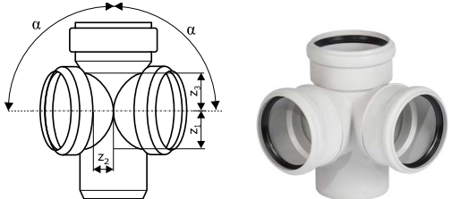
SKED – крестовина двухплоскостная 87°
