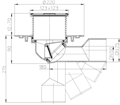
Рис. 1. Трап для балконов и террас HL80.
