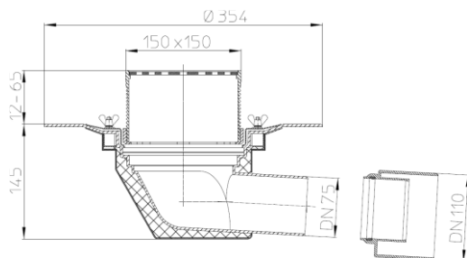
Рис. 1. Кровельная воронка HL64B.
