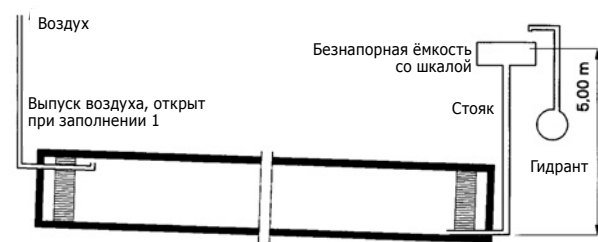
Рис. 10 Проверка герметичности
