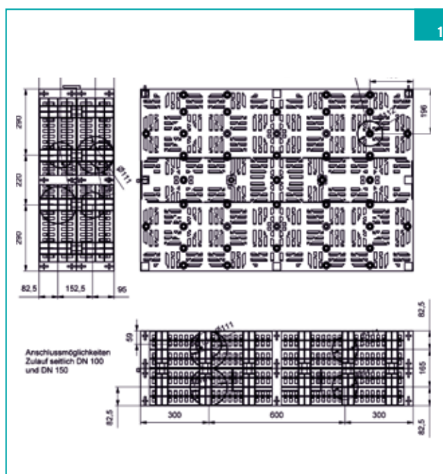
1 ■ Боковая проекция DRAINFIX BLOC
