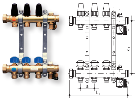
Коллектор для тёплого пола (с расходомером)
