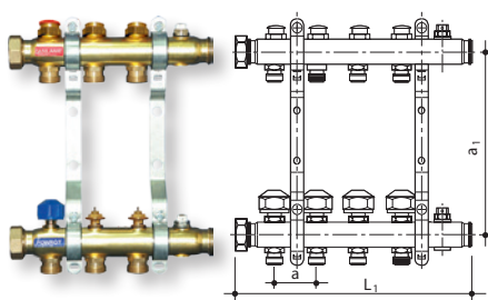
Коллектор для тёплого пола (без расходомера)
