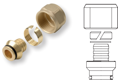
Соединитель для трубы PE-Xc
