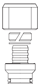
Соединитель для труб PE-RT/Al/PE-RT, PE-Xc
