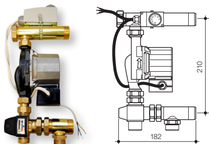
Смесительный узел с трехходовым клапаном
