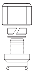
Соединитель для трубы PE-RT/Al/PE-RT
