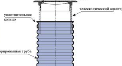
Люк B125 или D400 с телескопическим адаптером
