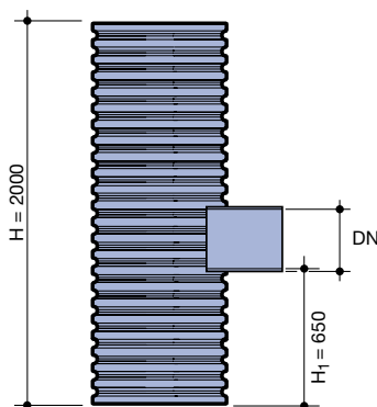
DN 600, DN 425 колодец, заглушенный на заводе Объем отстойника устанавливается на заводе Выходной патрубок dn 200 SWrk для DN 600 и 425, а также dn 160 SWrk для соединения с системой из гладкостенных труб гк – гладкий конец
