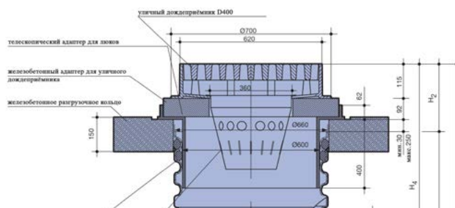
Уличный дождеприёмник или дождеприёмник из серого чугуна на телескопическом адаптере
