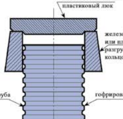
Полимерный или железобетонный люк, установленный на конической горловине
