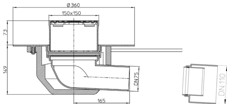
Рис. 1. Кровельная воронка HL64.1BP.
