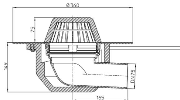
Рис. 1. Кровельная воронка HL64.1F/7.
