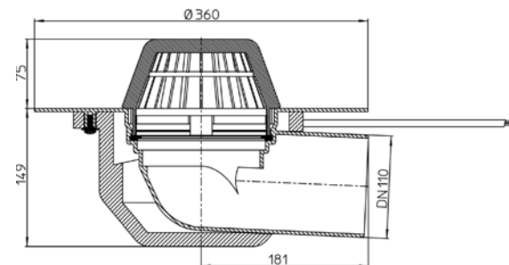
Рис. 2. Кровельная воронка HL64.1F/1.
