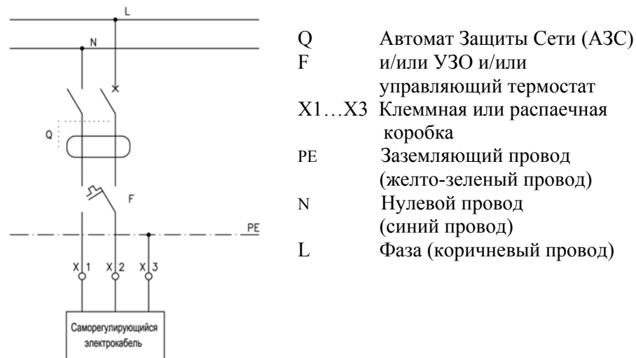
Рис. 5. Схема подключения электрообогрева кровельной воронки HL64.1F к электрической сети.
